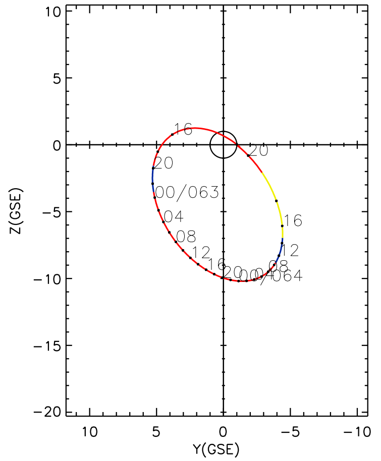
CLUSTER 2 orbit 2010 062 (03/03) 13:56 UT to 2010 064 (03/05) 20:16 UT
