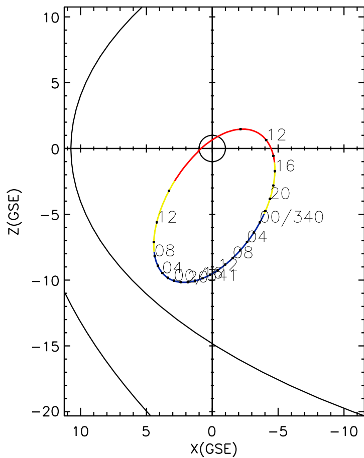
CLUSTER 2 orbit 2009 339 (12/05) 09:01 UT to 2009 341 (12/07) 15:21 UT
