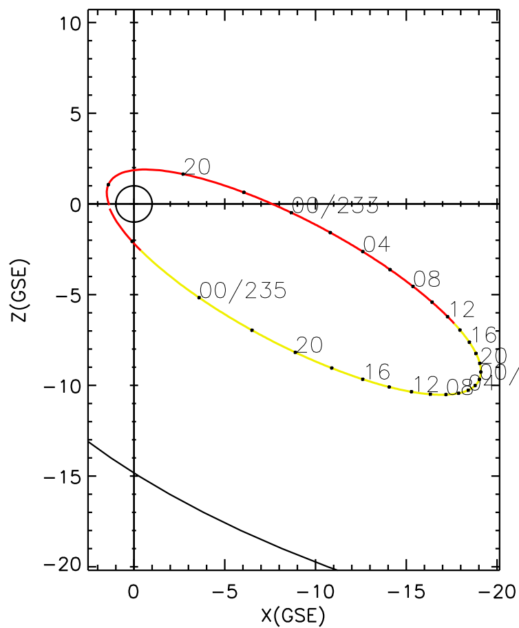
CLUSTER 2 orbit 2009 232 (08/20) 17:36 UT to 2009 235 (08/23) 02:41 UT
