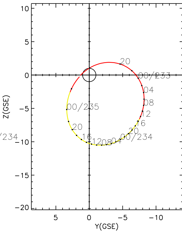
CLUSTER 2 orbit 2009 232 (08/20) 17:36 UT to 2009 235 (08/23) 02:41 UT
