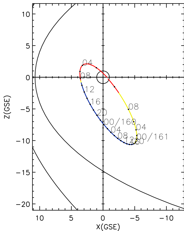
CLUSTER 2 orbit 2009 159 (06/08) 01:26 UT to 2009 161 (06/10) 10:26 UT
