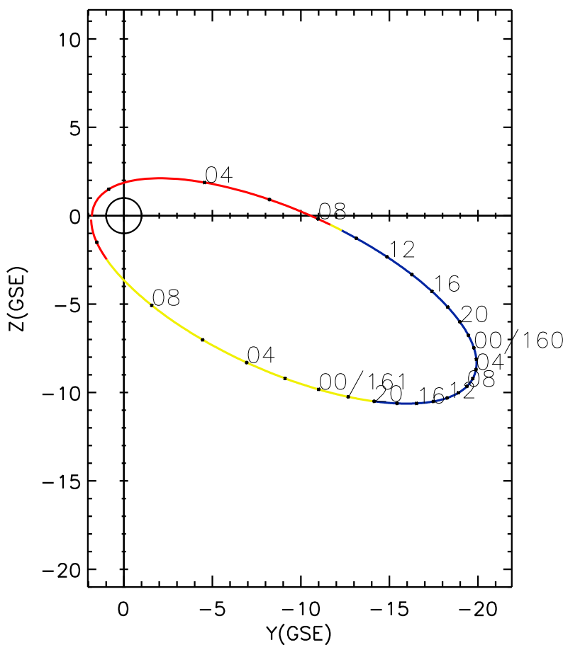
CLUSTER 2 orbit 2009 159 (06/08) 01:26 UT to 2009 161 (06/10) 10:26 UT
