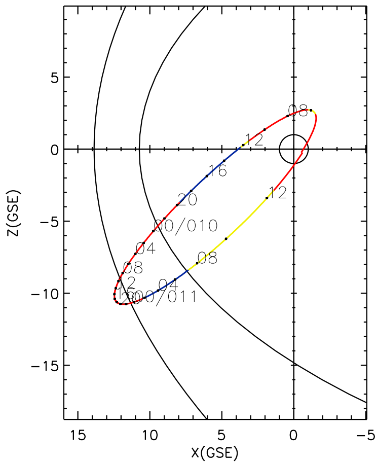
CLUSTER 2 orbit 2009 009 (01/09) 04:11 UT to 2009 011 (01/11) 13:16 UT
