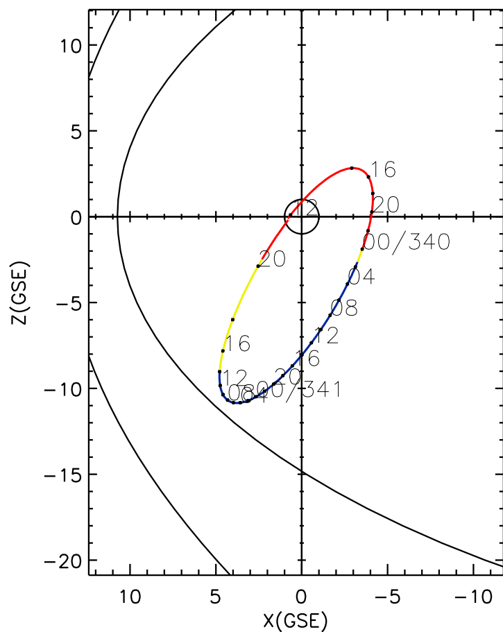
CLUSTER 2 orbit 2008 339 (12/04) 11:56 UT to 2008 341 (12/06) 21:01 UT
