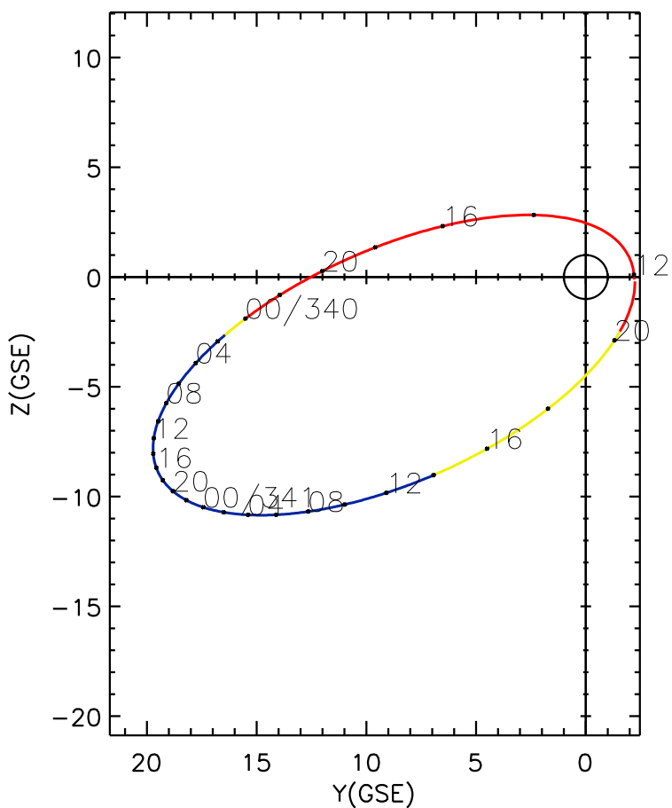
CLUSTER 2 orbit 2008 339 (12/04) 11:56 UT to 2008 341 (12/06) 21:01 UT
