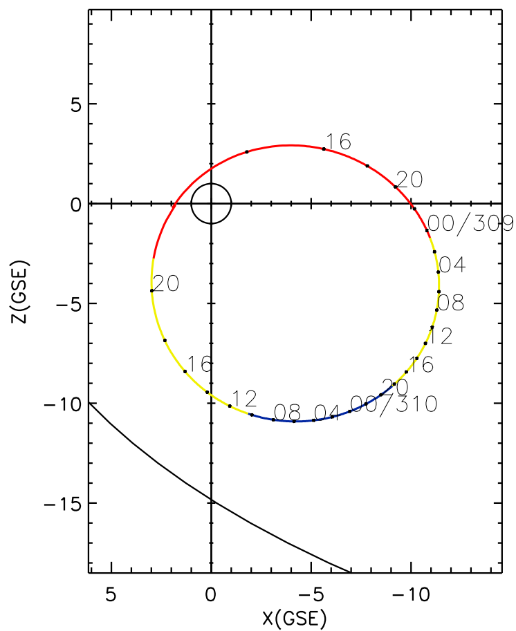
CLUSTER 2 orbit 2008 308 (11/03) 12:41 UT to 2008 310 (11/05) 21:51 UT
