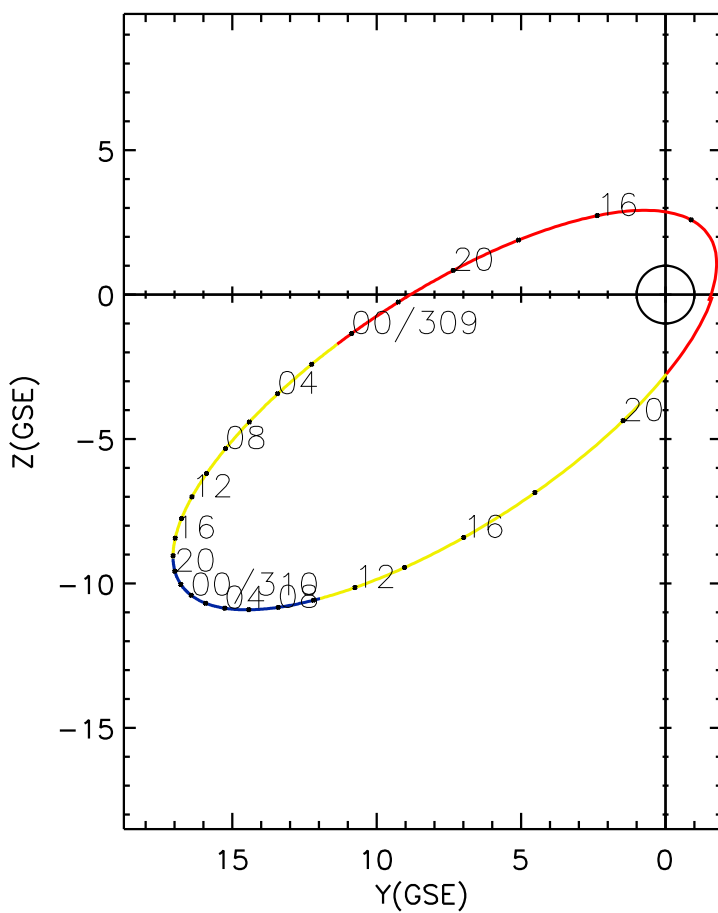
CLUSTER 2 orbit 2008 308 (11/03) 12:41 UT to 2008 310 (11/05) 21:51 UT
