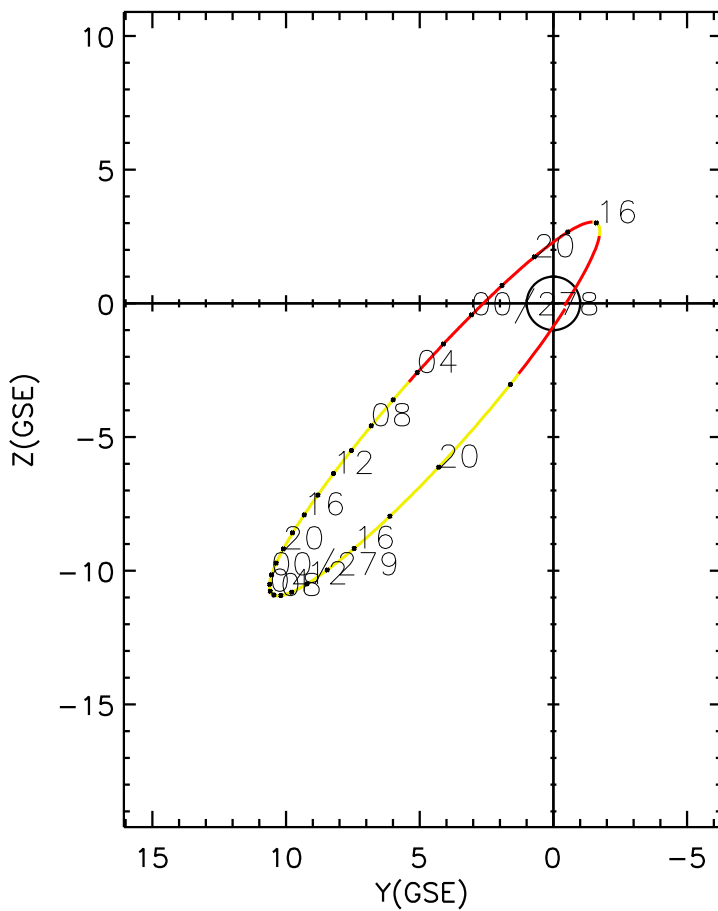
CLUSTER 2 orbit 2008 277 (10/03) 14:01 UT to 2008 279 (10/05) 23:06 UT
