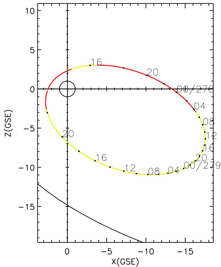
CLUSTER 2 orbit 2008 277 (10/03) 14:01 UT to 2008 279 (10/05) 23:06 UT
