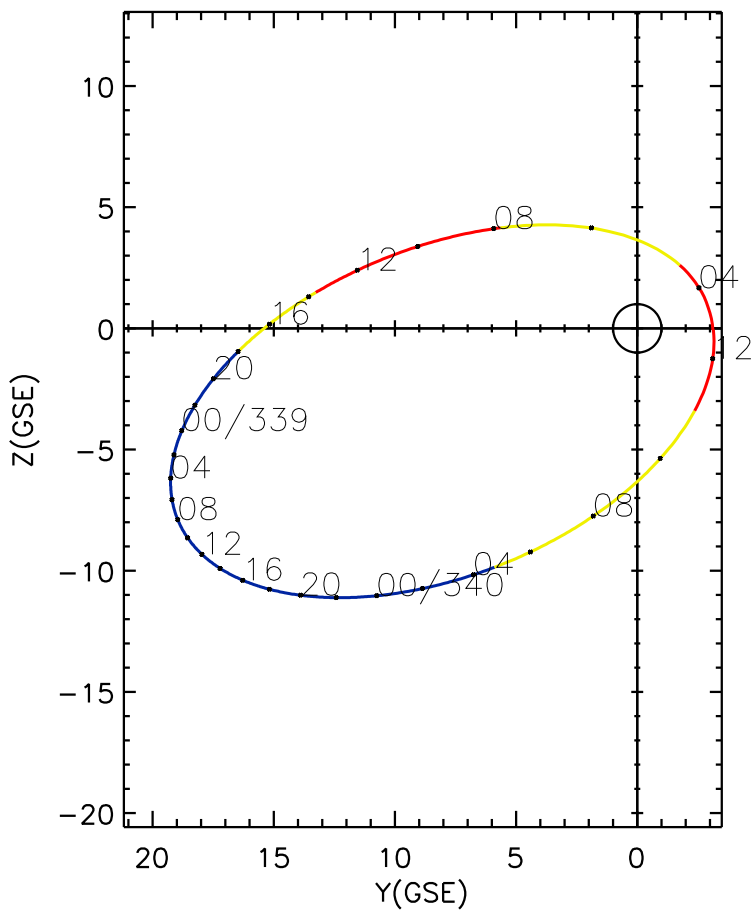
CLUSTER 2 orbit 2007 338 (12/04) 03:21 UT to 2007 340 (12/06) 12:26 UT
