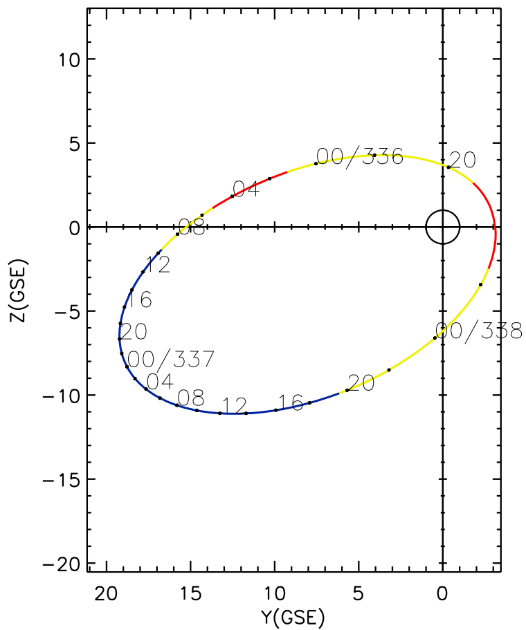
CLUSTER 2 orbit 2007 335 (12/01) 18:16 UT to 2007 338 (12/04) 03:21 UT
