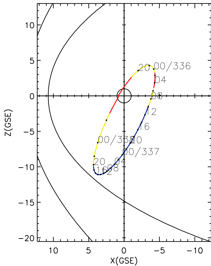
CLUSTER 2 orbit 2007 335 (12/01) 18:16 UT to 2007 338 (12/04) 03:21 UT
