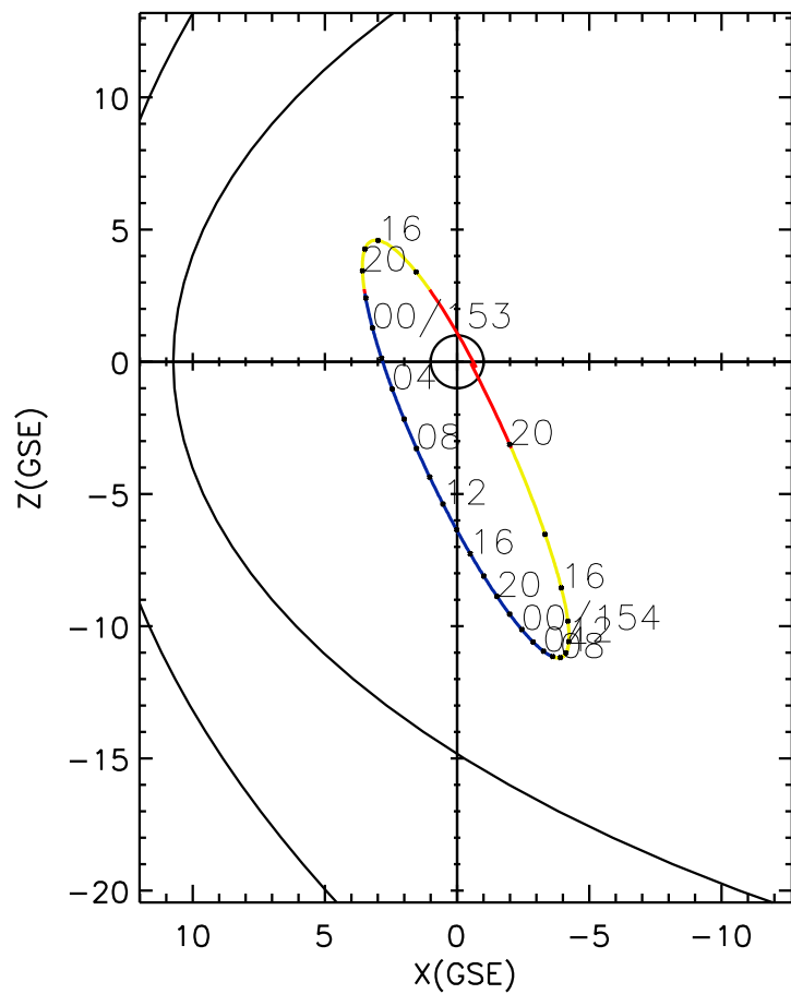
CLUSTER 2 orbit 2007 152 (06/01) 12:26 UT to 2007 154 (06/03) 21:11 UT
