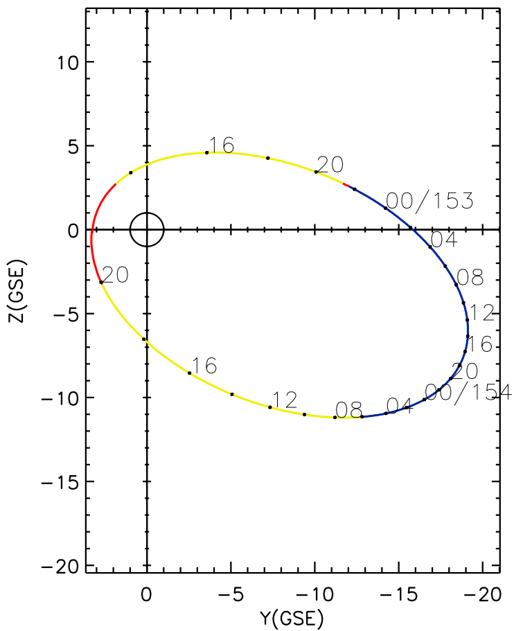
CLUSTER 2 orbit 2007 152 (06/01) 12:26 UT to 2007 154 (06/03) 21:11 UT
