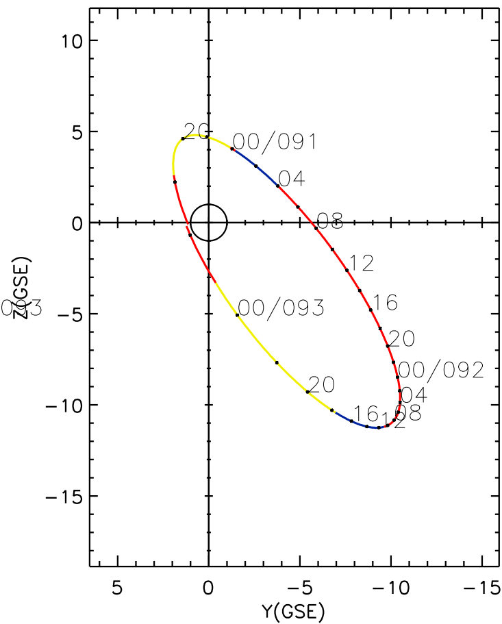
CLUSTER 2 orbit 2007 090 (03/31) 17:06 UT to 2007 093 (04/03) 02:11 UT
