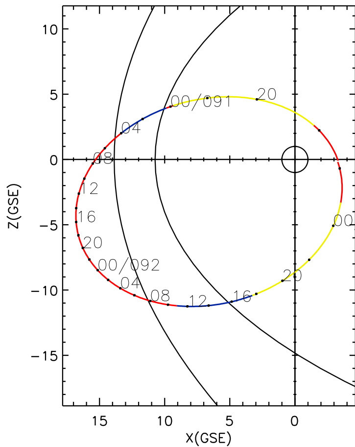
CLUSTER 2 orbit 2007 090 (03/31) 17:06 UT to 2007 093 (04/03) 02:11 UT
