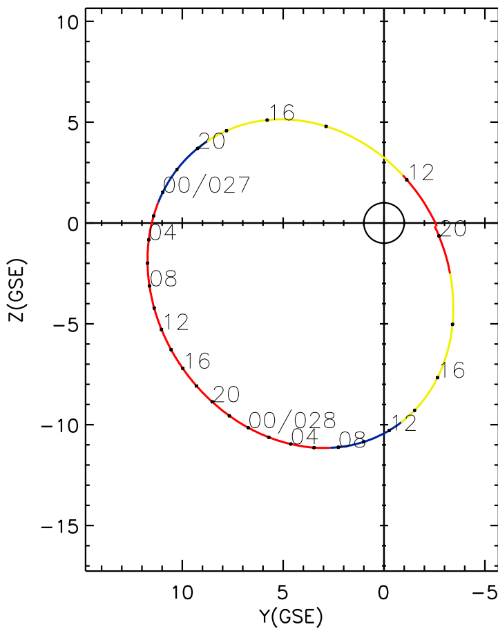
CLUSTER 2 orbit 2007 026 (01/26) 11:06 UT to 2007 028 (01/28) 20:11 UT
