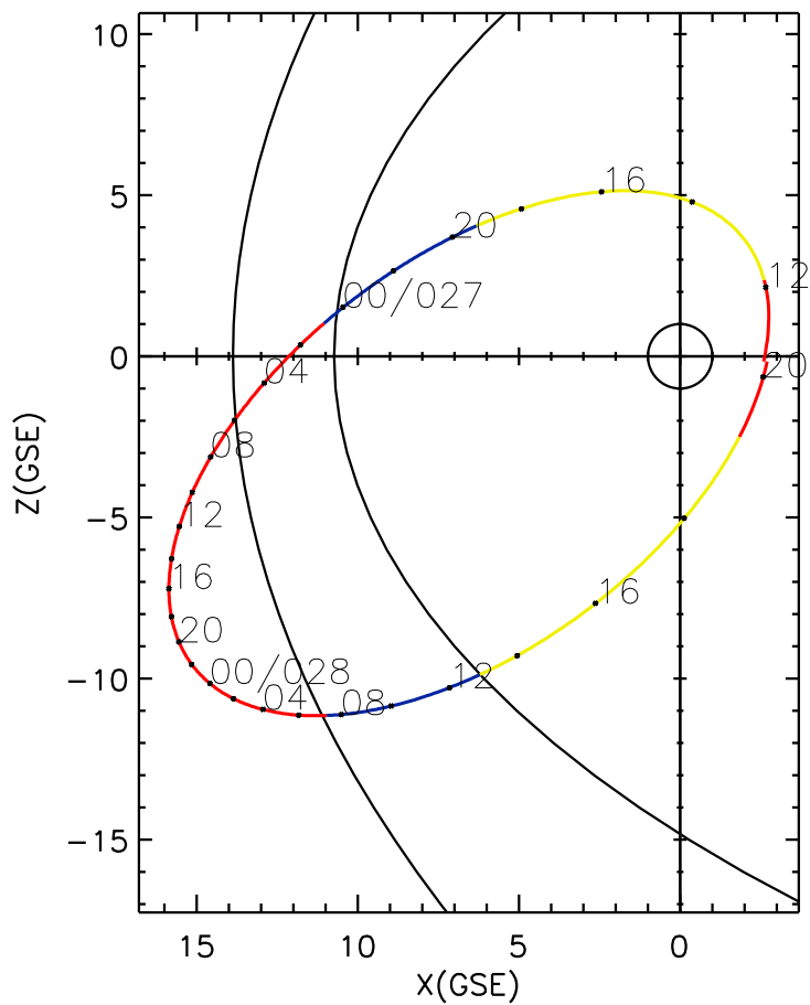
CLUSTER 2 orbit 2007 026 (01/26) 11:06 UT to 2007 028 (01/28) 20:11 UT
