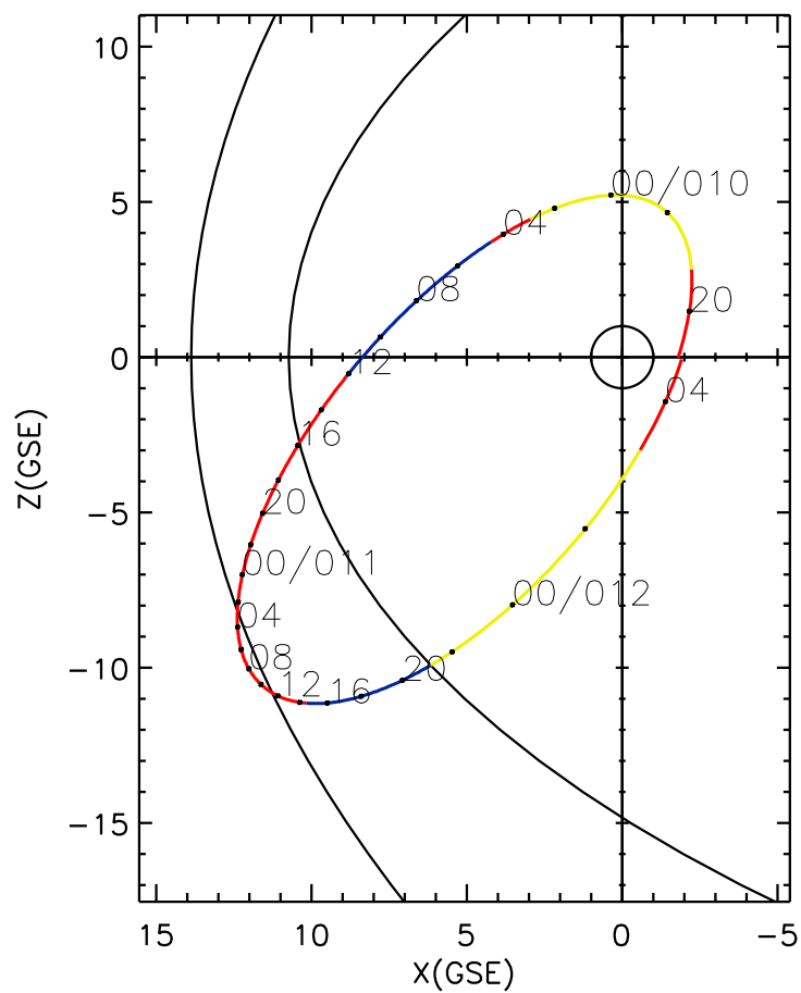
CLUSTER 2 orbit 2007 009 (01/09) 19:26 UT to 2007 012 (01/12) 04:31 UT
