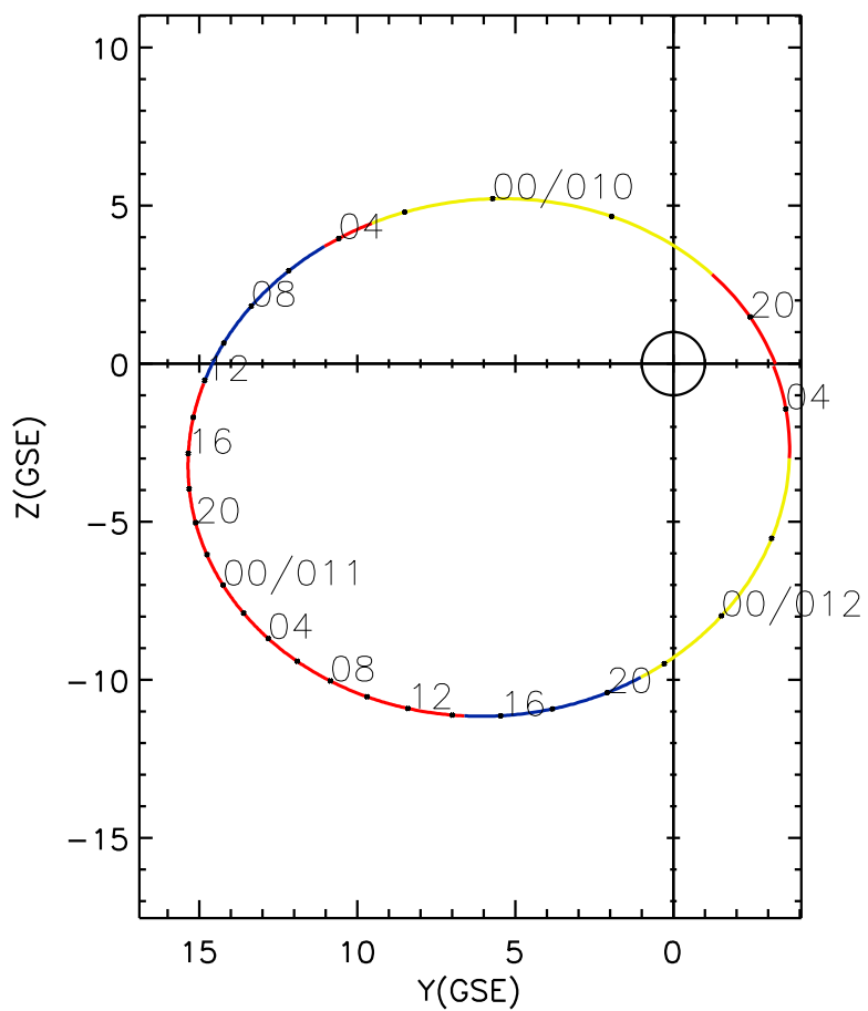
CLUSTER 2 orbit 2007 009 (01/09) 19:26 UT to 2007 012 (01/12) 04:31 UT
