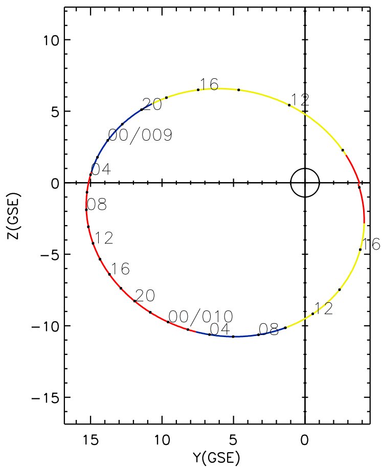
CLUSTER 2 orbit 2006 008 (01/08) 09:01 UT to 2006 010 (01/10) 18:06 UT
