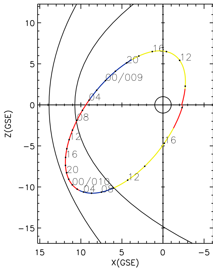
CLUSTER 2 orbit 2006 008 (01/08) 09:01 UT to 2006 010 (01/10) 18:06 UT
