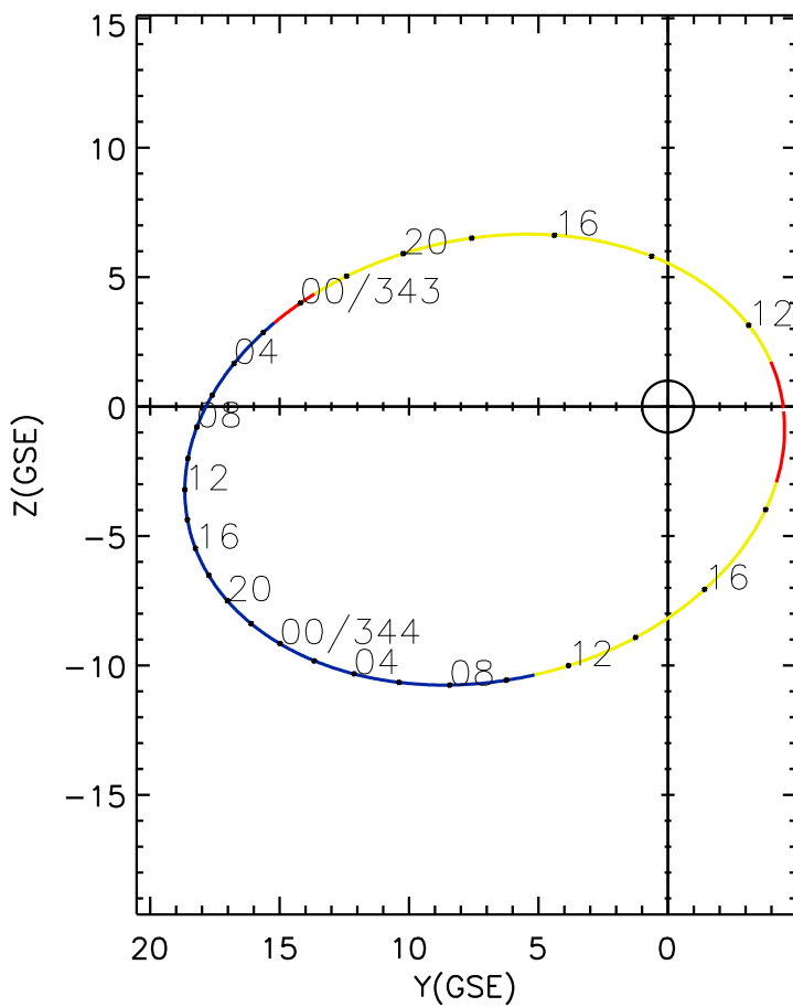
CLUSTER 2 orbit 2005 342 (12/08) 10:36 UT to 2005 344 (12/10) 19:41 UT
