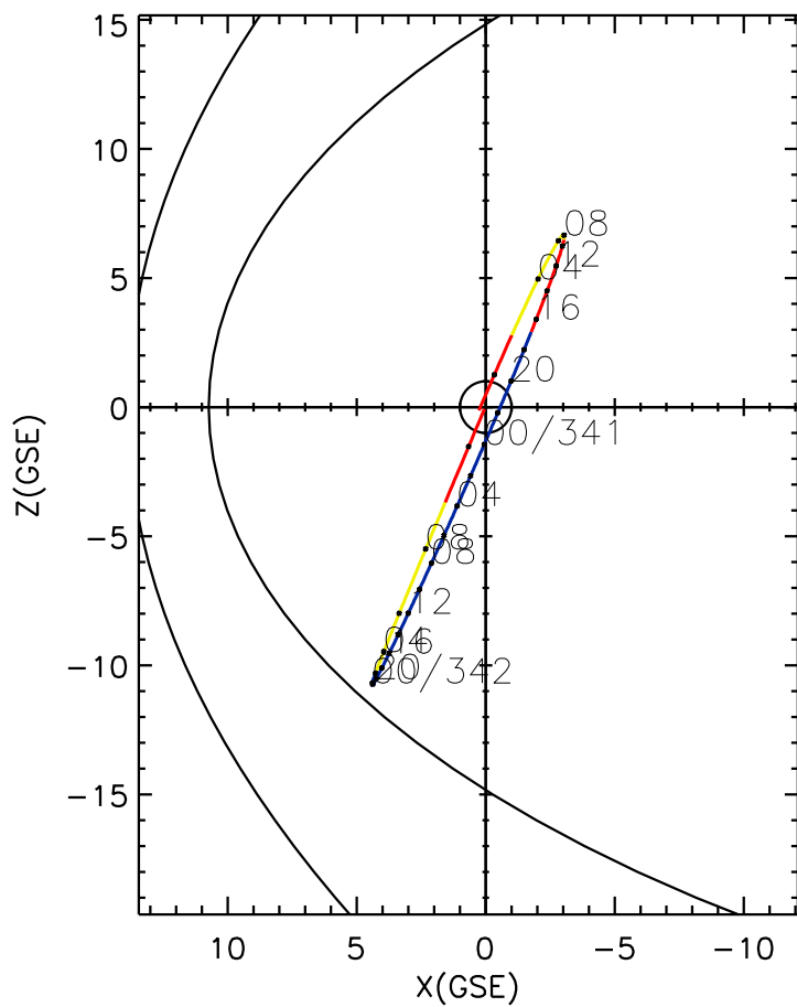
CLUSTER 2 orbit 2005 340 (12/06) 01:26 UT to 2005 342 (12/08) 10:36 UT
