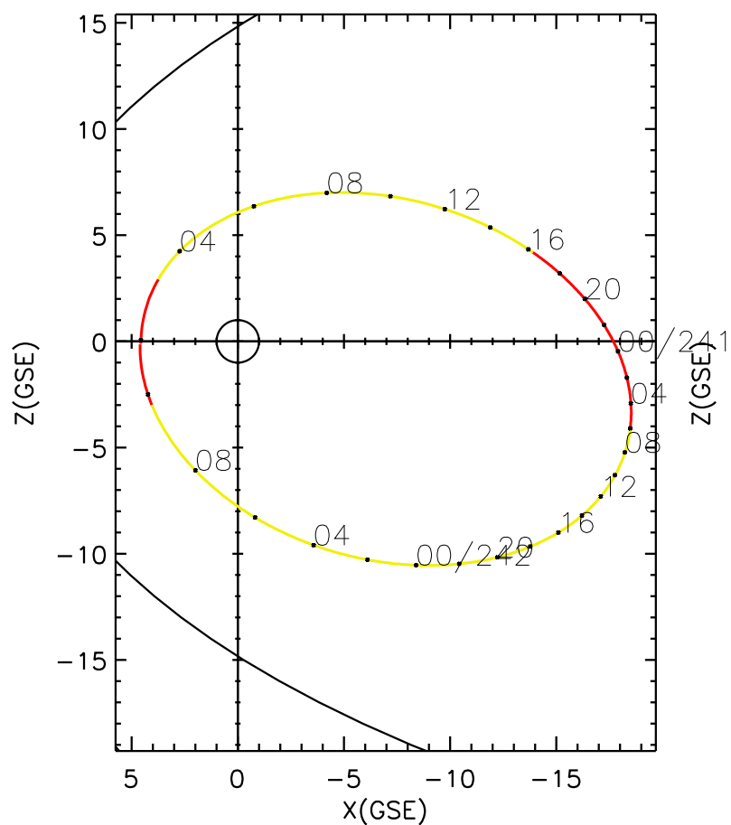
CLUSTER 2 orbit 2005 240 (08/28) 01:56 UT to 2005 242 (08/30) 11:01 UT
