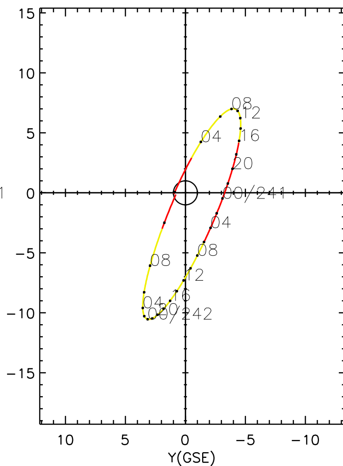
CLUSTER 2 orbit 2005 240 (08/28) 01:56 UT to 2005 242 (08/30) 11:01 UT
