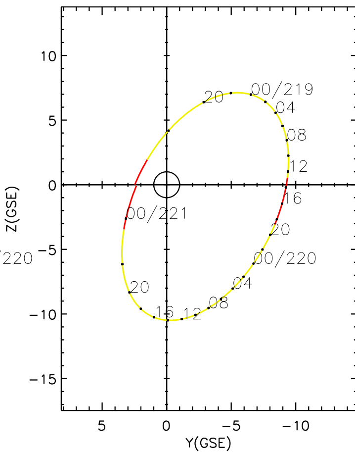
CLUSTER 2 orbit 2005 218 (08/06) 16:01 UT to 2005 221 (08/09) 01:06 UT
