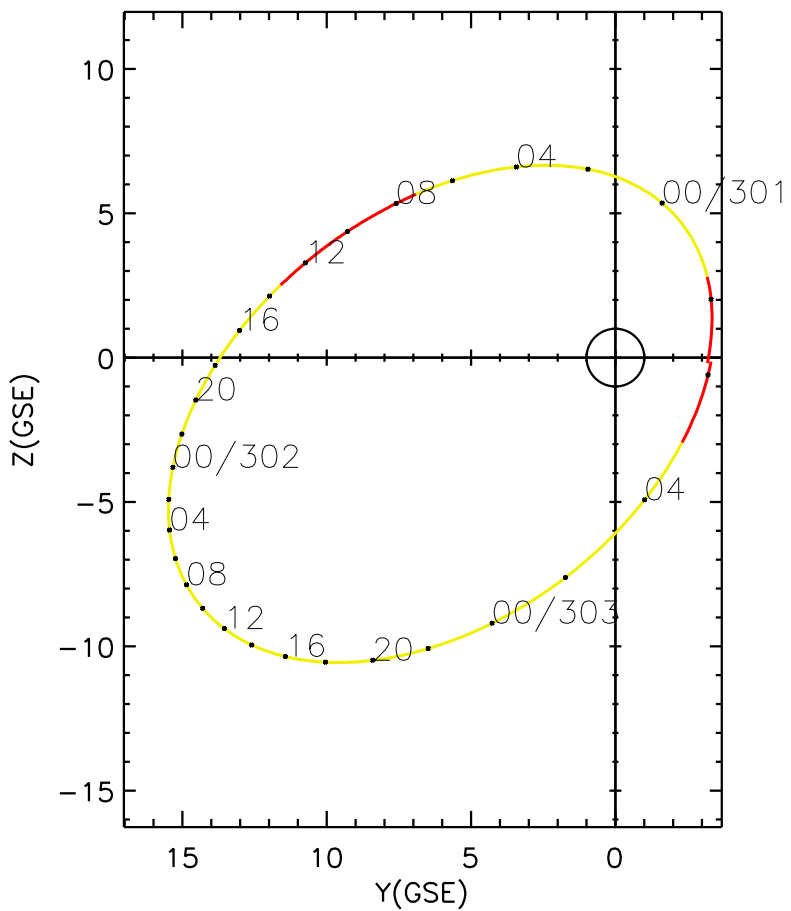
CLUSTER 2 orbit 2004 300 (10/26) 21:06 UT to 2004 303 (10/29) 06:11 UT
