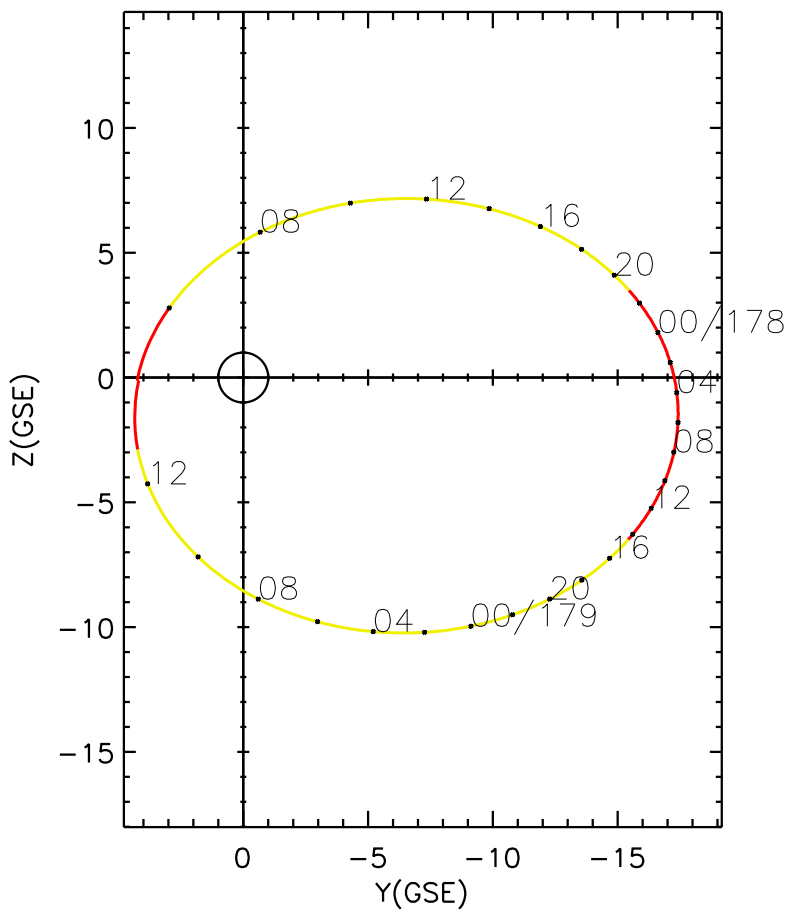
CLUSTER 2 orbit 2004 177 (06/25) 04:46 UT to 2004 179 (06/27) 13:51 UT
