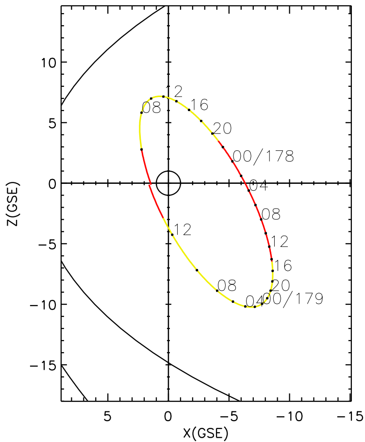
CLUSTER 2 orbit 2004 177 (06/25) 04:46 UT to 2004 179 (06/27) 13:51 UT
