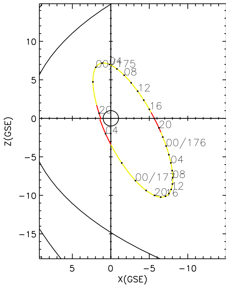
CLUSTER 2 orbit 2004 174 (06/22) 19:41 UT to 2004 177 (06/25) 04:46 UT
