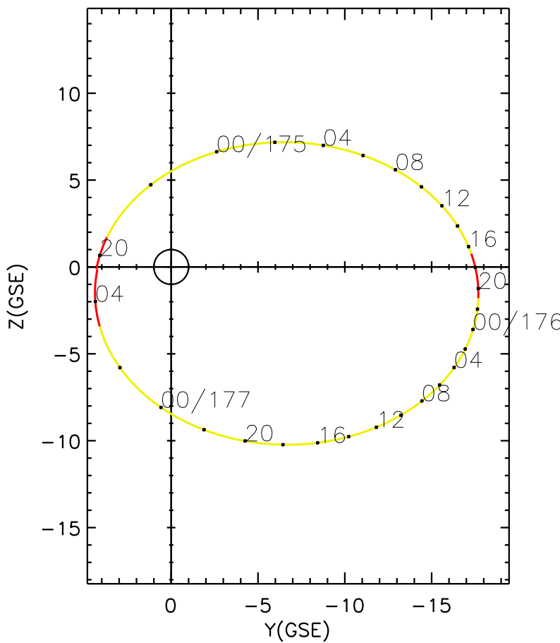
CLUSTER 2 orbit 2004 174 (06/22) 19:41 UT to 2004 177 (06/25) 04:46 UT
