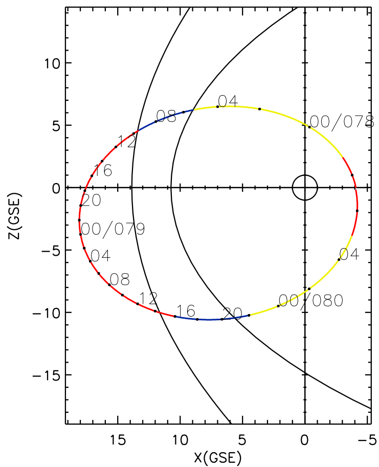
CLUSTER 2 orbit 2004 077 (03/17) 21:36 UT to 2004 080 (03/20) 06:41 UT
