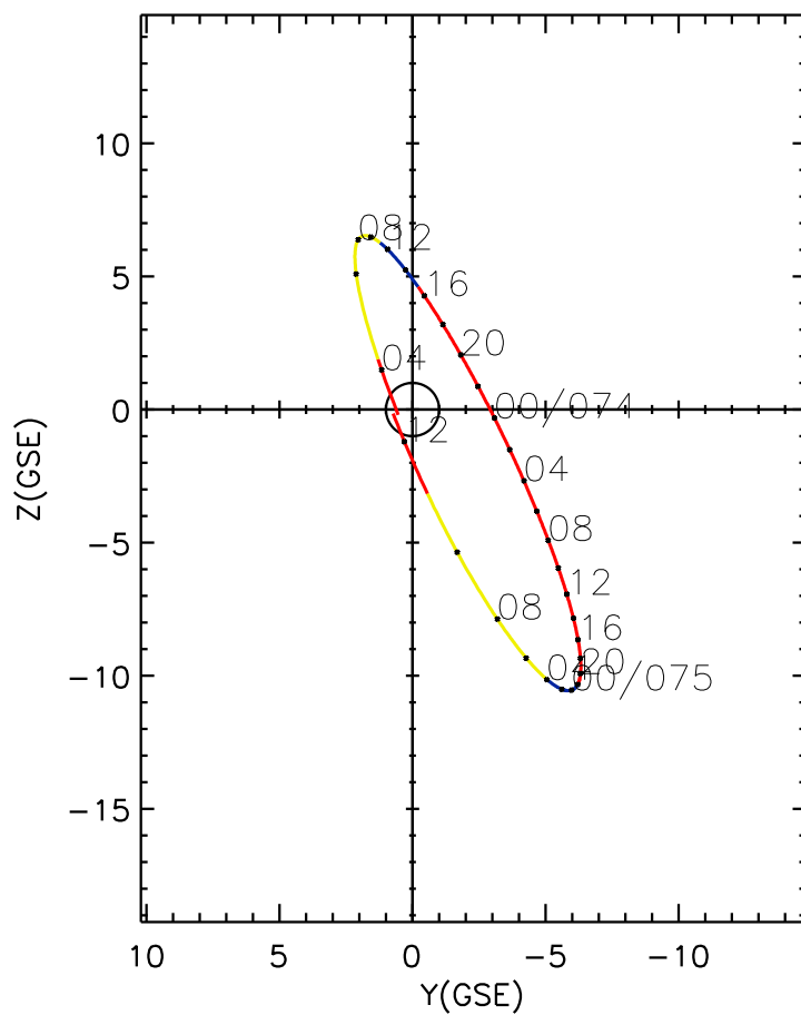
CLUSTER 2 orbit 2004 073 (03/13) 03:20 UT to 2004 075 (03/15) 12:25 UT
