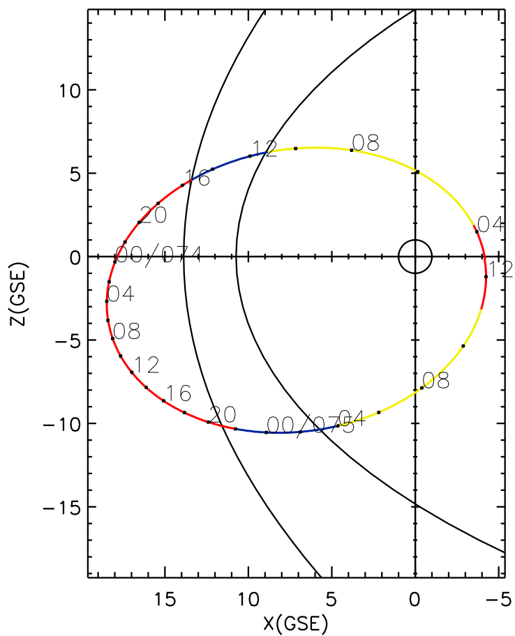
CLUSTER 2 orbit 2004 073 (03/13) 03:20 UT to 2004 075 (03/15) 12:25 UT
