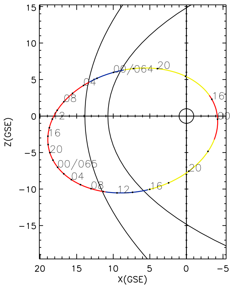
CLUSTER 2 orbit 2004 063 (03/03) 15:00 UT to 2004 066 (03/06) 00:10 UT
