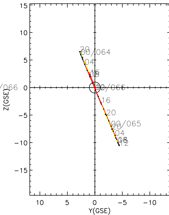
CLUSTER 2 orbit 2004 063 (03/03) 15:00 UT to 2004 066 (03/06) 00:10 UT
