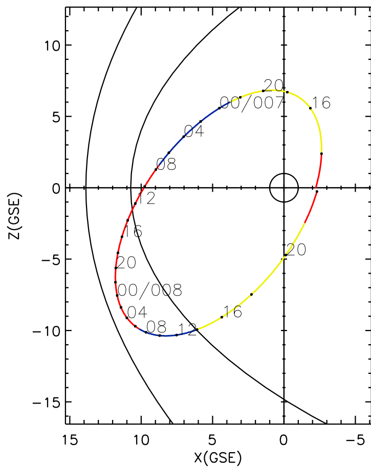
CLUSTER 2 orbit 2004 006 (01/06) 13:01 UT to 2004 008 (01/08) 22:01 UT
