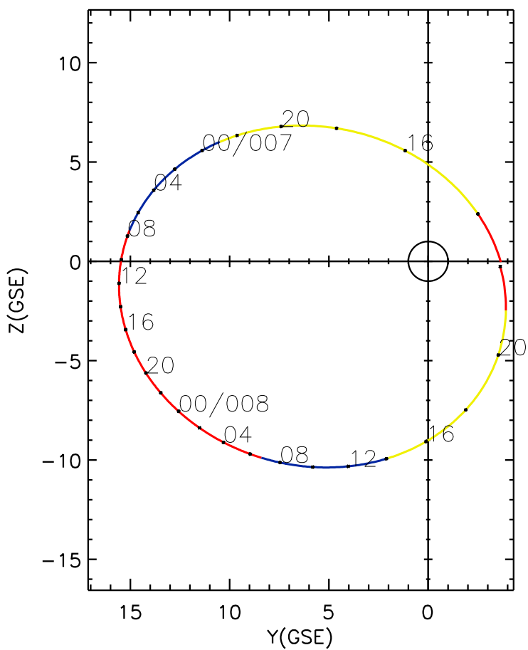
CLUSTER 2 orbit 2004 006 (01/06) 13:01 UT to 2004 008 (01/08) 22:01 UT
