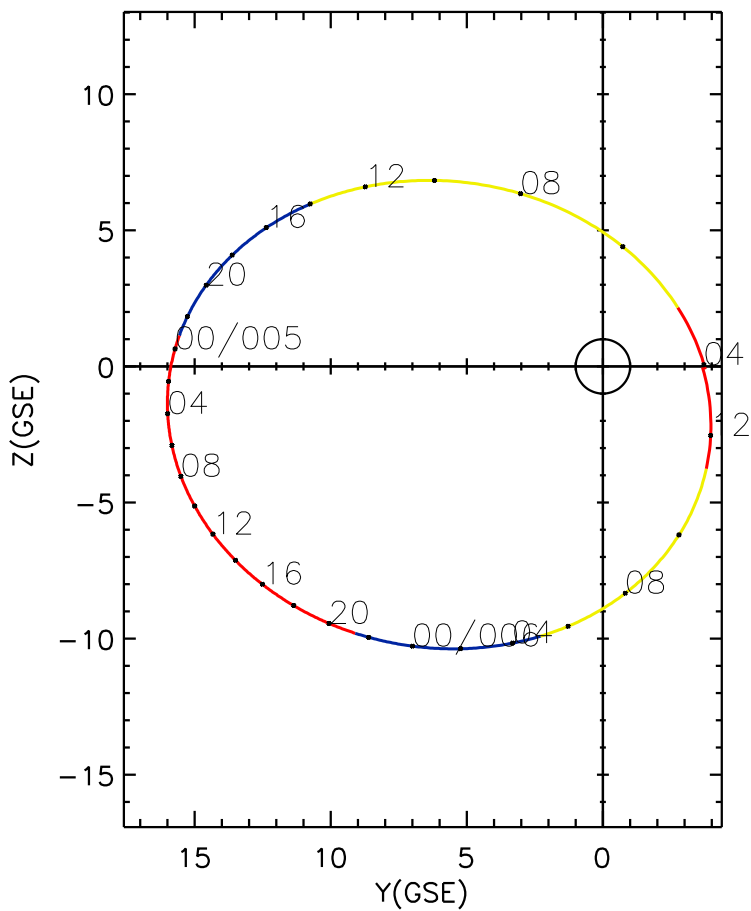
CLUSTER 2 orbit 2004 004 (01/04) 03:56 UT to 2004 006 (01/06) 13:01 UT
