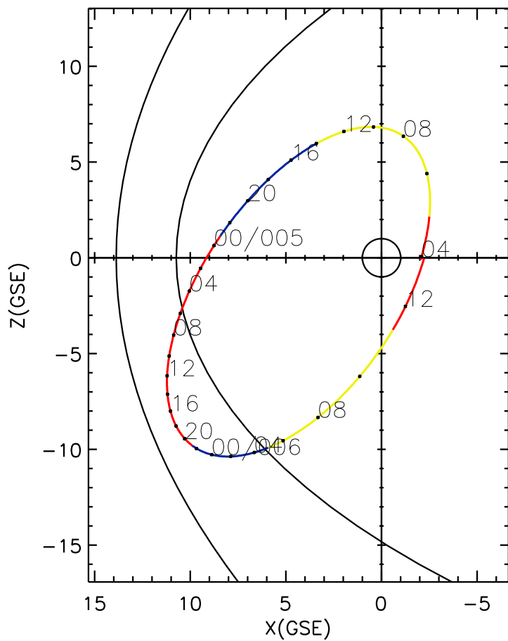
CLUSTER 2 orbit 2004 004 (01/04) 03:56 UT to 2004 006 (01/06) 13:01 UT
