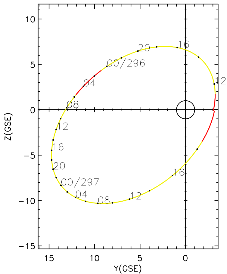
CLUSTER 2 orbit 2003 295 (10/22) 10:46 UT to 2003 297 (10/24) 19:51 UT
