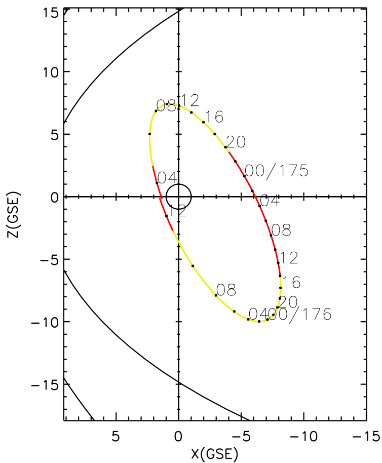
CLUSTER 2 orbit 2003 174 (06/23) 03:30 UT to 2003 176 (06/25) 12:35 UT
