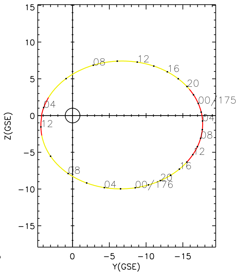
CLUSTER 2 orbit 2003 174 (06/23) 03:30 UT to 2003 176 (06/25) 12:35 UT
