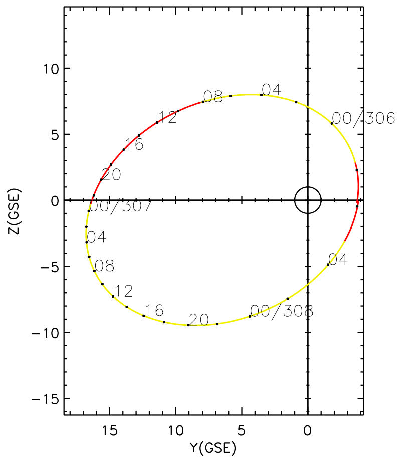
CLUSTER 2 orbit 2002 305 (11/01) 21:00 UT to 2002 308 (11/04) 06:10 UT
