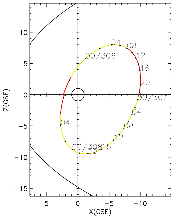
CLUSTER 2 orbit 2002 305 (11/01) 21:00 UT to 2002 308 (11/04) 06:10 UT
